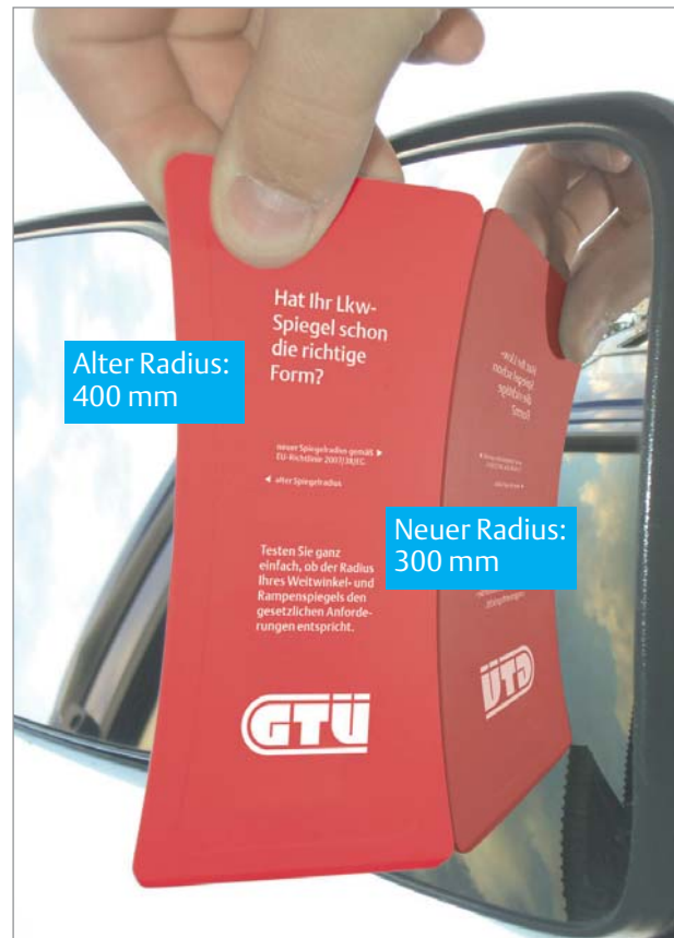
Halten Sie die Schablone senkrecht auf das Spiegelglas. Passt die Seite mit dem Radius 300 mm ohne Spalt auf das Glas, sind bereits die neuen Spiegelgläser montiert.
